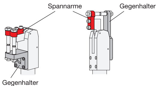
Spannbacken
