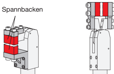
Gegenhalter
